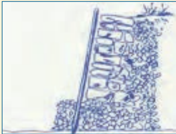
Stützmauer
